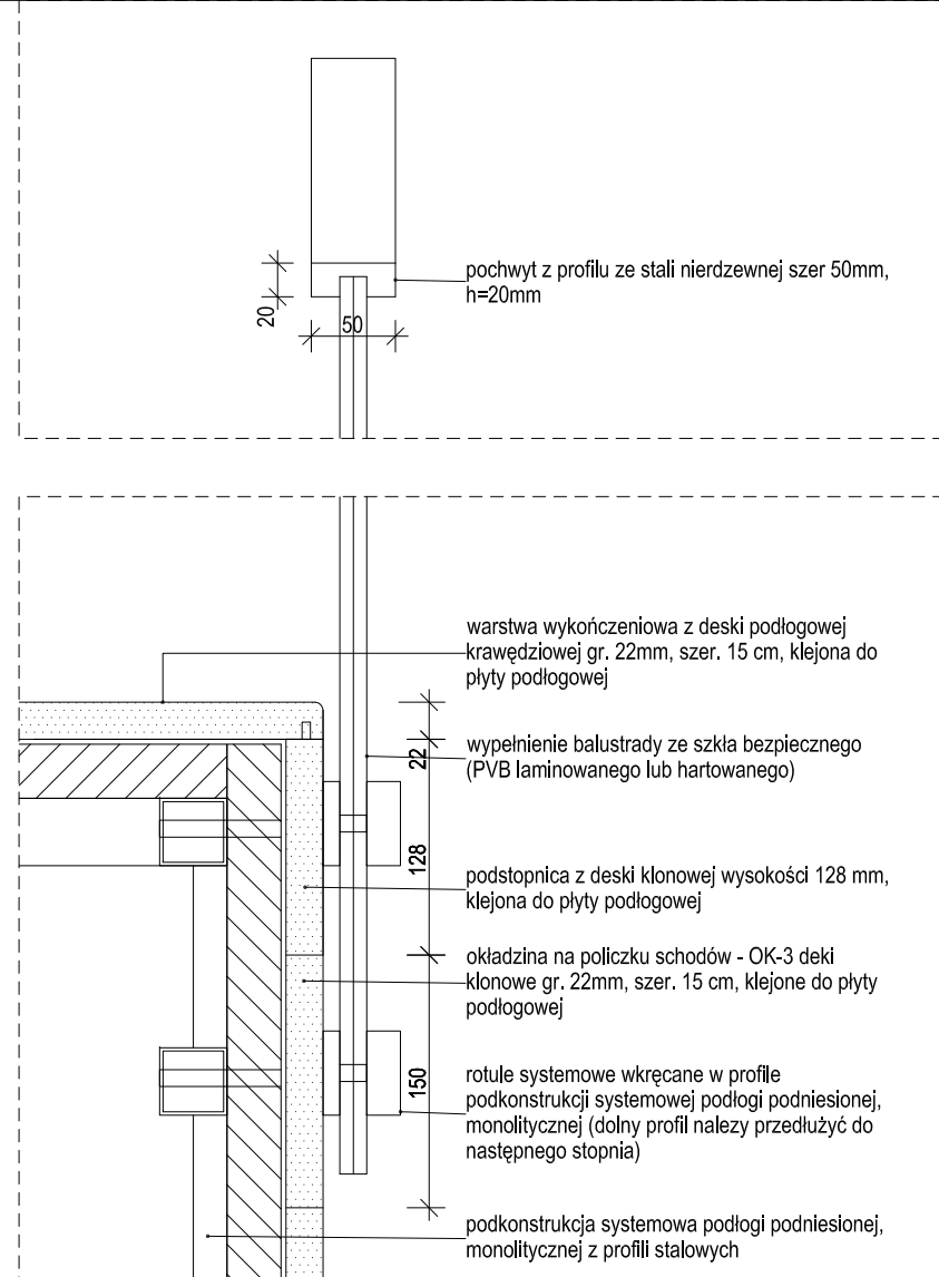
Detal skala 1:5 - mocowanie balustrady do półeczka schodów
