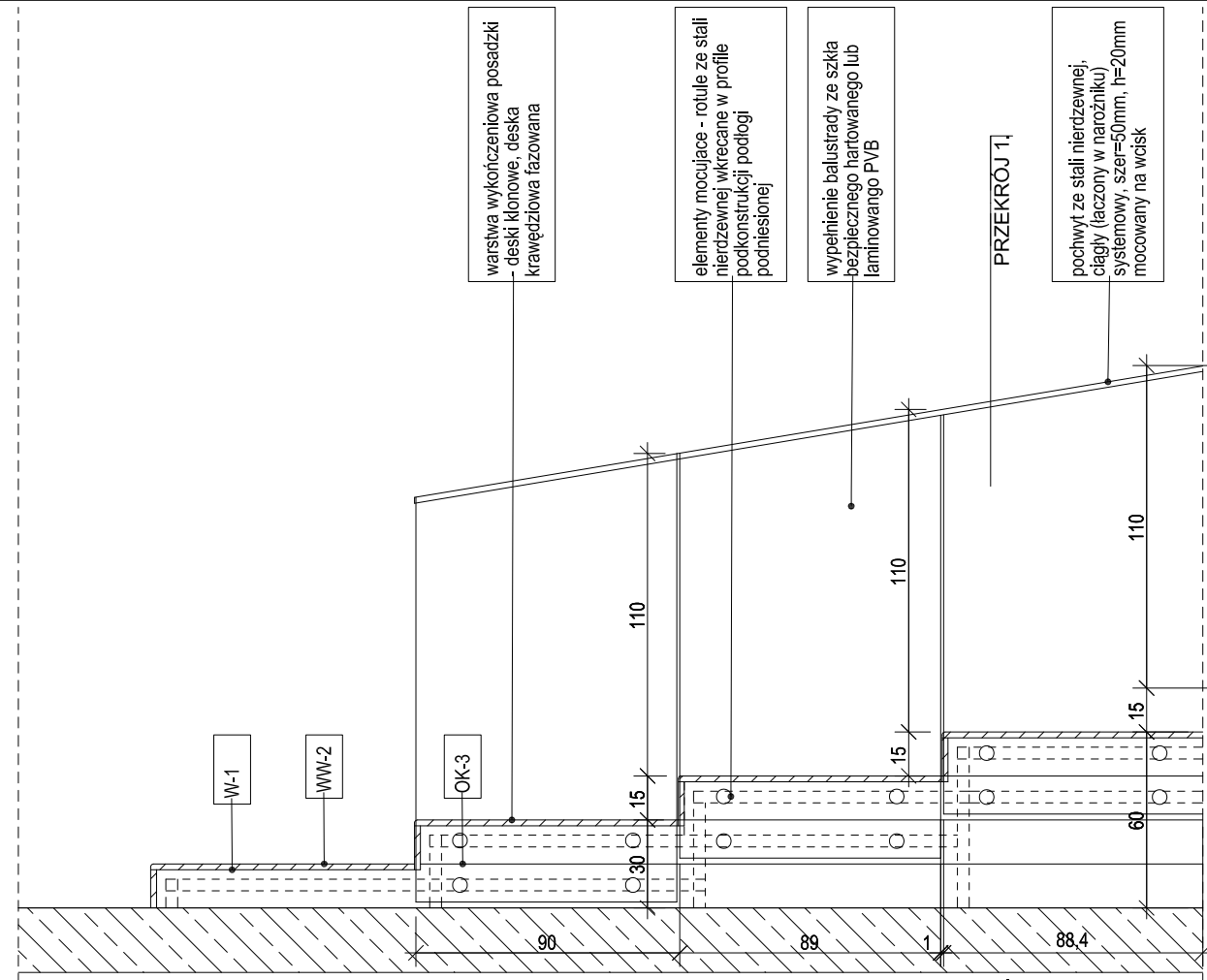
WIDOK 1.1.
