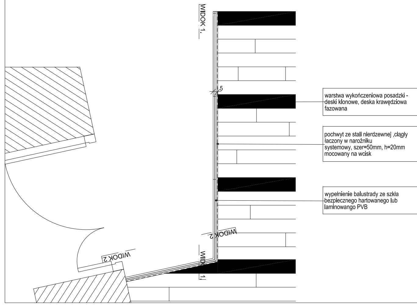
PRZEKRÓJ 1.1.
