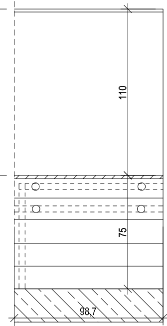
WIDOK 2.2.
