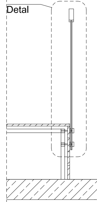
PRZEKRÓJ 1.1.
