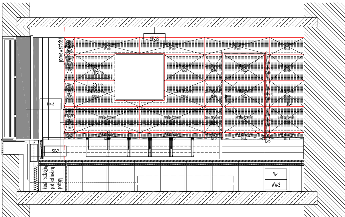
GEOMETRIA OKŁADZINY Z PANELI CEMENTOWO-WIÓROWYCH OK-1.1b
