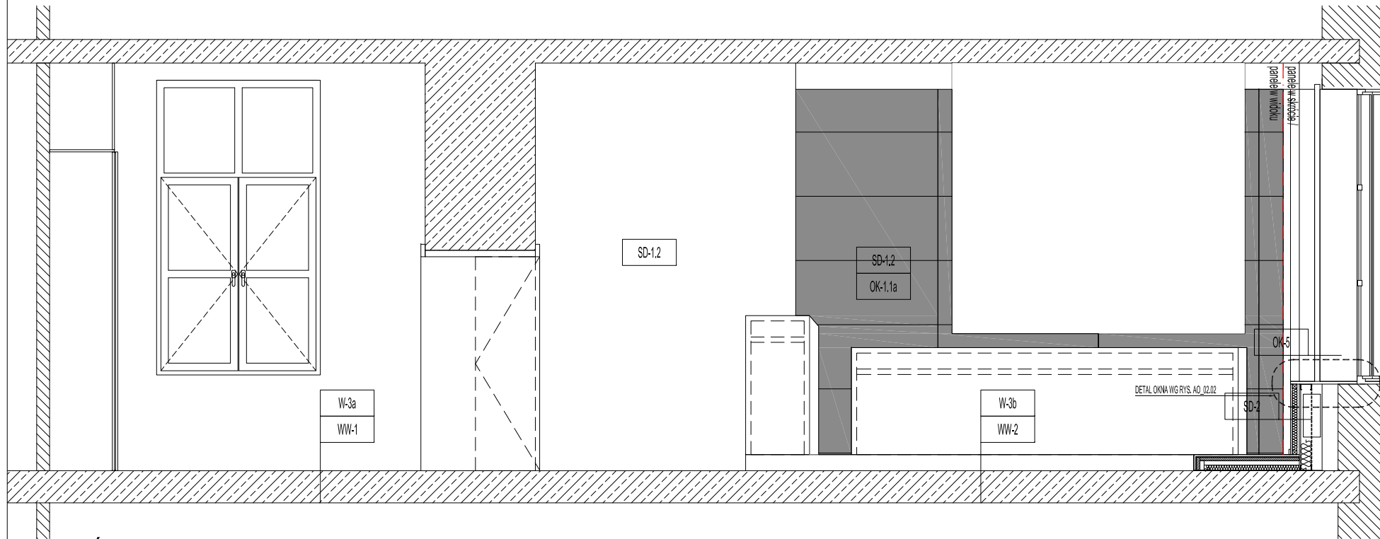
WIDOK ŚCIANY 2-2
