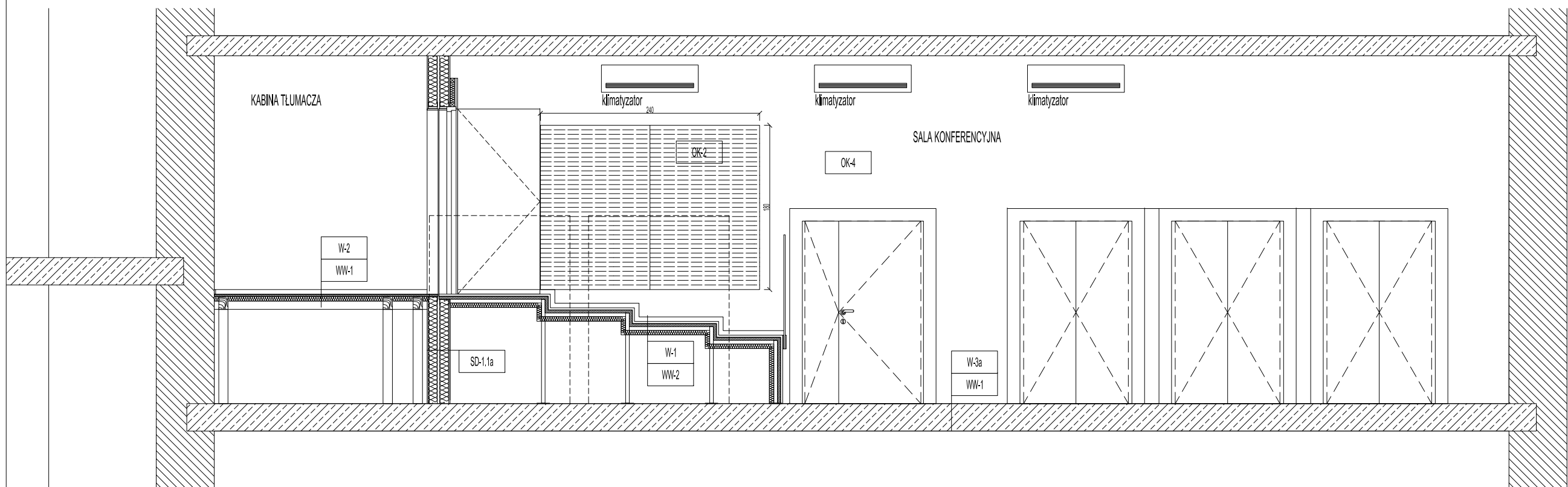
WIDOK ŚCIANY 5-5
